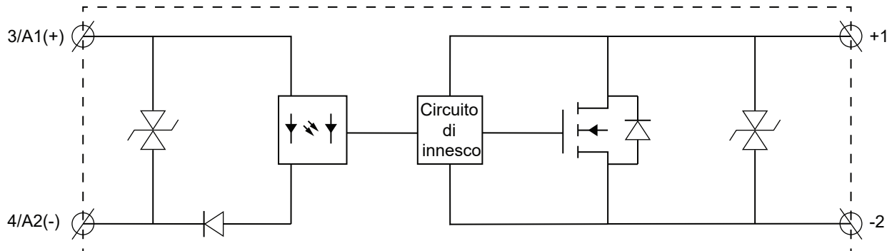
Fig. 11 Schema funzionale RM1D
