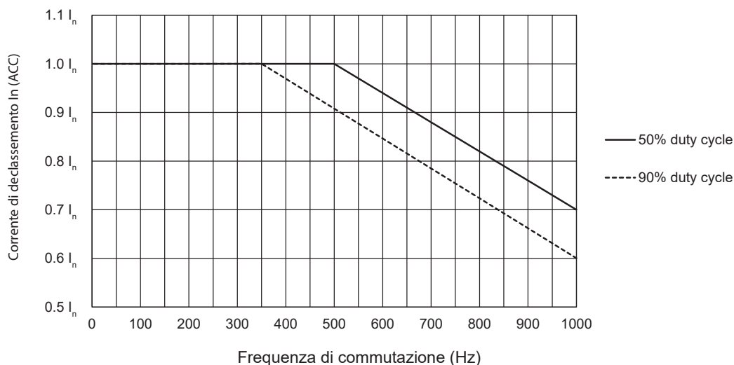
Fig. 4 Corrente di declassamento vs. frequenza di commutazione
