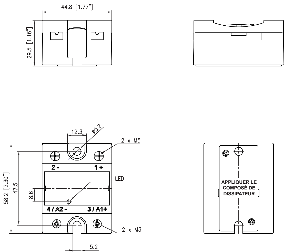
Fig. 1 Dimensions RM1D
